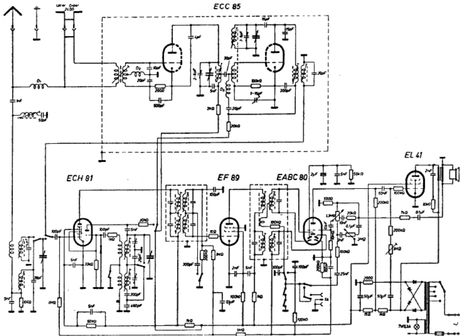
CONTINENTAL (Continental-Rundfunk GmbH, Osterode, Harz) - Mod. Imperial 250 - Ricevitore a modulazione di ampiezza e di frequenza. Onde lunghe da 140 a 375 kc/s, onde medie da 510 a 1700 kc/s, onde ultracorte FM da 87,5 a 100,5 Mc/s. Commutazione di gamma e di accensione con quattro tasti. Altoparlante ellittico. Resa di uscita 2 watt. Prod. 1956.
